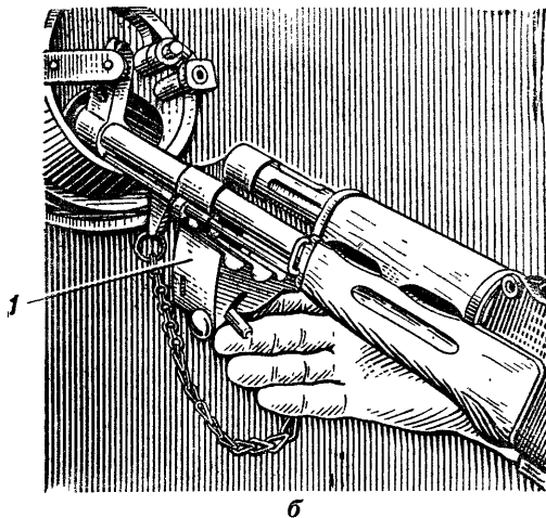
Рис. 89. Установка автомата в бойницу: а — отделение замка от бойницы; б — присоединение замка к автомату; 1 — бойница; 2 — замок; 3 — планка
