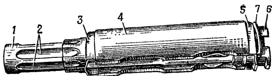
Рис. 40. Газовая трубка со ствольной накладкой: 1 — газовая трубка; 2 — направляющие ребра для газового поршня; 3 — передняя соединительная муфта; 4 — ствольная накладка; 5 — задняя соединительная муфта; 6 — выступ; 7 — пластинчатая пружина
