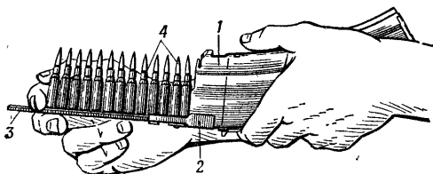
Рис. 63. Снаряжение магазина патронами из обоймы:
