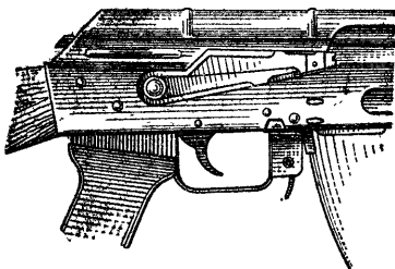
Рис. 61. Автомат (пулемет) поставлен на предохранитель
