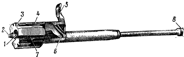
Рис. 37. Затворная рама с газовым поршнем:
