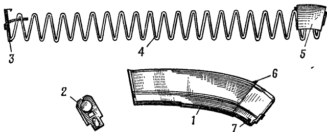
Рис. 43. Магазин:
