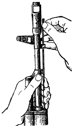
Рис. 5. Отделение шомпола
