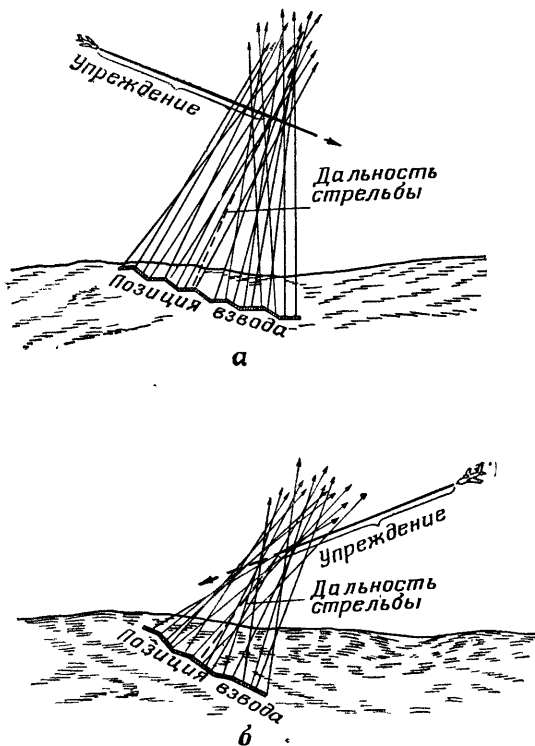
Рис. 95. Ведение огня заградительным способом по самолету:
