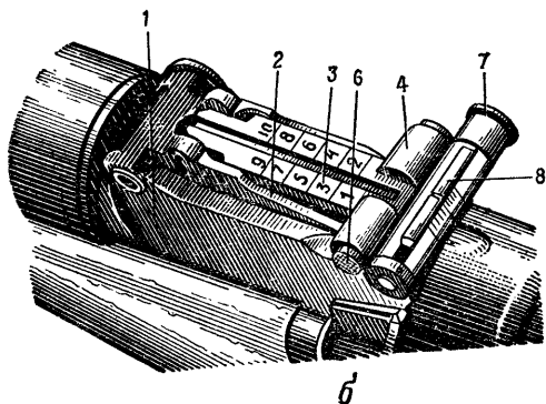
Рис. 31. Прицел:
