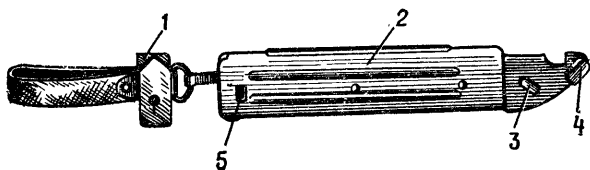
Рис. 45. Ножны:
