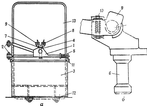
Рис. 100. Шкворневая установка для стрельбы через входную дверь:
