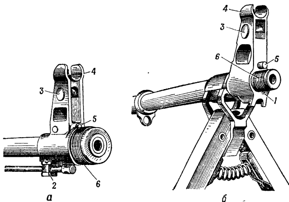
Рис. 29. Основание мушки:
