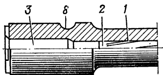
Рис. 27. Ствол:
