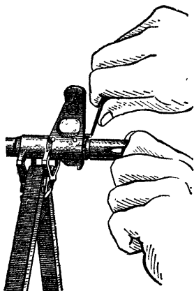
Рис. 6. Отделение пламегасителя
