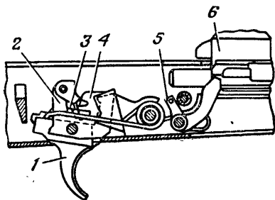
Рис. 51. Положение частей ударно-спускового механизма после выстрела при переводчике, установленном на одиночный огонь:
