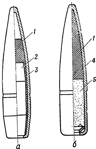
Рис. 48. Пули:
