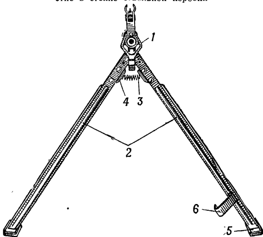
Рис. 36. Сошка пулемета:
