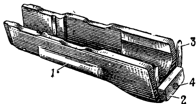
Рис. 42. Цевье (деревянное):
