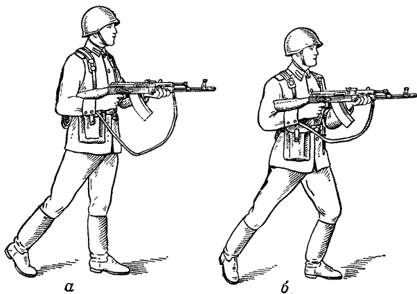
Рис. 83. Положение при стрельбе на ходу:
