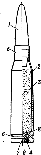
Рис. 47. Боевой патрон:
