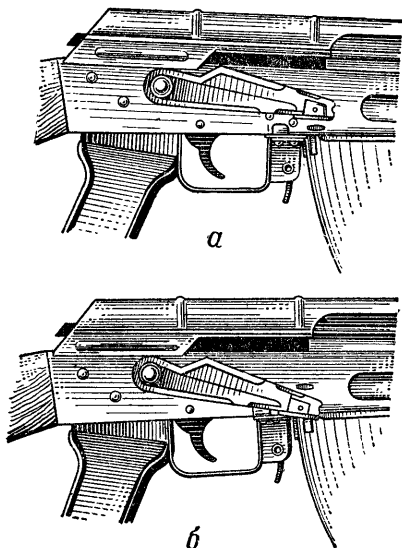
Рис. 68. Установка переводчика на необходимый вид огня:
