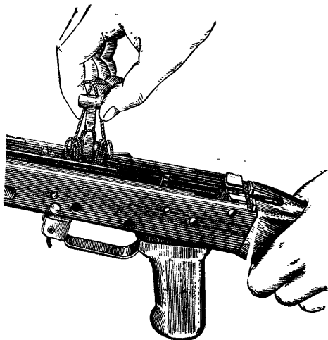
Рис. 18. Вынимание трубчатой оси
