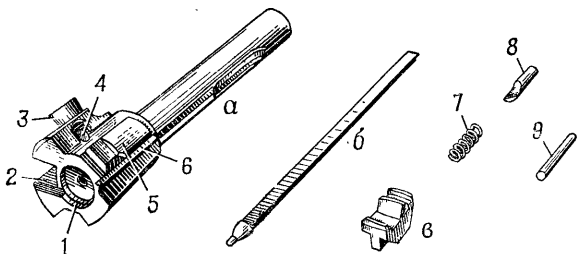
Рис. 38. Затвор:
