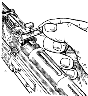
Рис. 67. Установка целика
