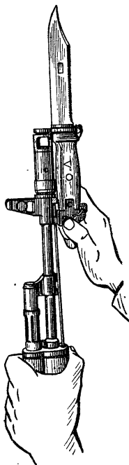
Рис. 26. Отмыка- ние штыка-ножа
