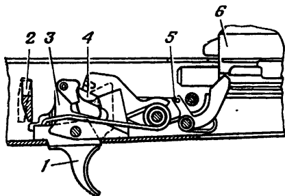
Рис. 50. Положение частей ударно-спускового механизма перед выстрелом: 1 — спусковой крючок; 2 — сектор переводчика; 3 — замедлитель курка; 4 — курок; 5 — шептало автоспуска; 6 — затворная рама
