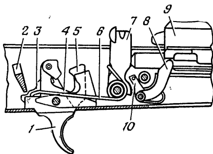
Рис. 49. Положение частей ударно-спускового механизма до заряжания при включенном предохранителе и спущенном курке:
