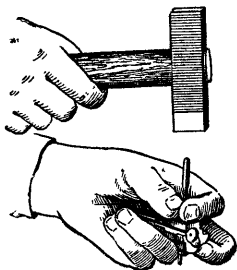
Рис. 16. Выталкивание шпильки при отделении выбрасывателя и ударника от затвора
