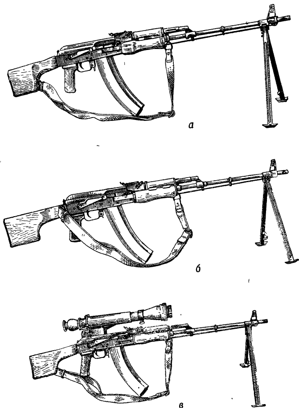
Рис. 2. Общий вид 5,45-мм ручного пулемета Калашникова:
