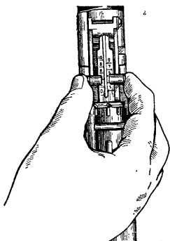
Рис. 66. Установка прицела
