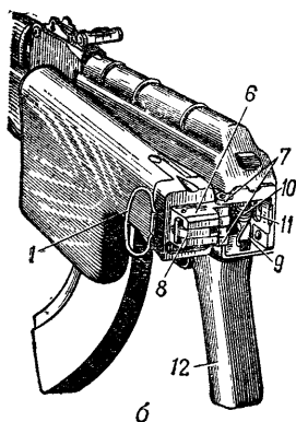
Рис. 34. Приклад и пистолетная рукоятка пулемета: а — постоянный приклад (в разрезе); б — складывающийся приклад (в сложенном положении); 1 — антабка для ремня; 2 — гнездо для принадлежности; 3 — затыльник; 4 — крышка; 5 — пружина для выталкивания пенала принадлежности; 6 — выступ приклада с ушками; 7 — проушина ствольной коробки; 8 — правая защелка приклада с пружиной; 9 — задняя часть левой защелки с насечкой; 10 — пружина защелки; 11 — вырез для правой защелки приклада; 12 — пистолетная рукоятка
